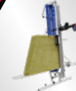
Isolatiemateriaal snijden met de accu-gloedraad-snijmachine van SPEWE
