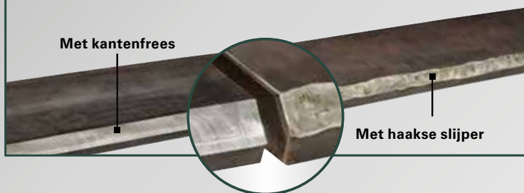
Materiaal: constructiestaal (S235JR) afgeschuinde kant 15 mm x 45°
